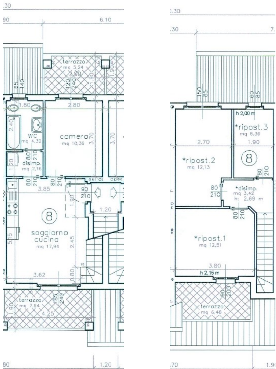
Estratto dagli atti di fabbrica – piano primo e piano sottotetto
