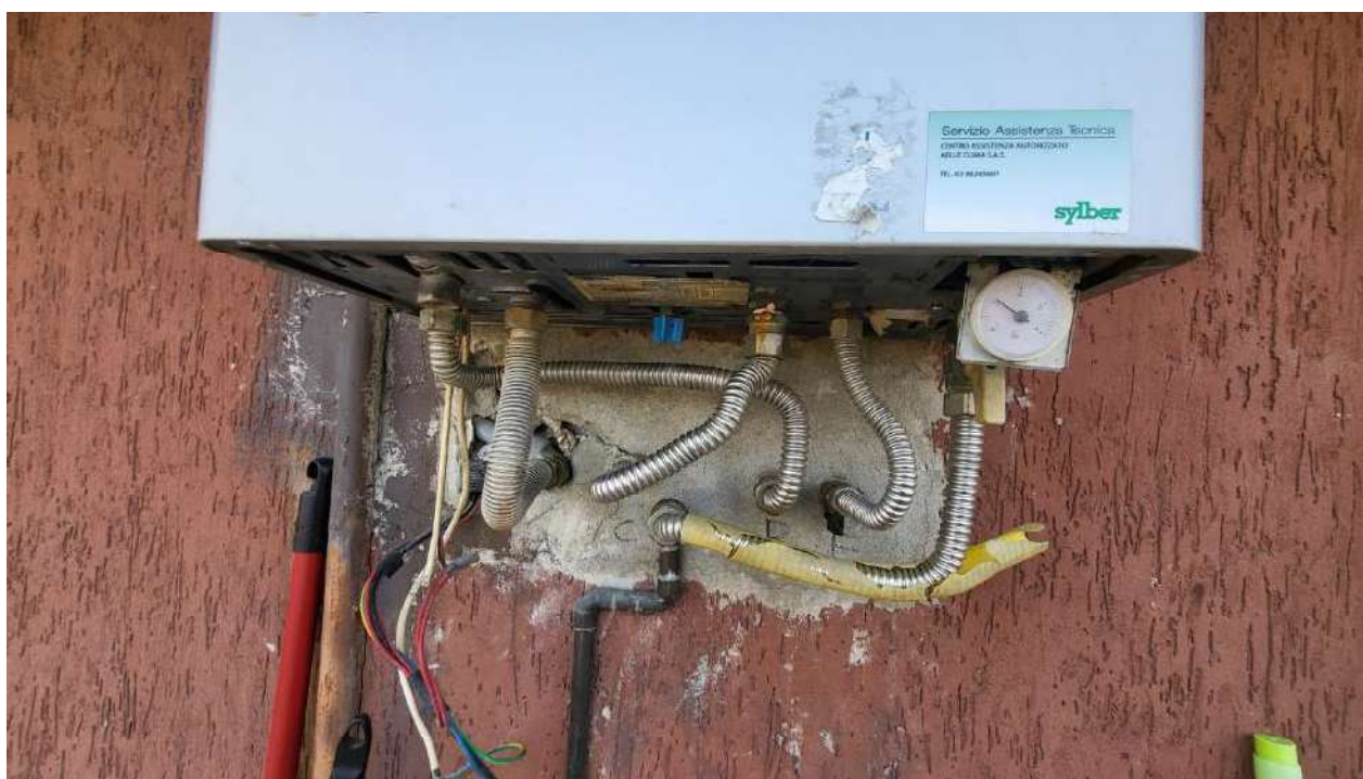
Dettagli – Fili elettrici della caldaia murale autonoma a gas metano
