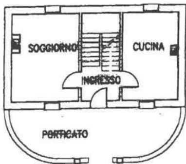
PIANTA PIANO TERRA H= 2.63 SCALA 1:200
