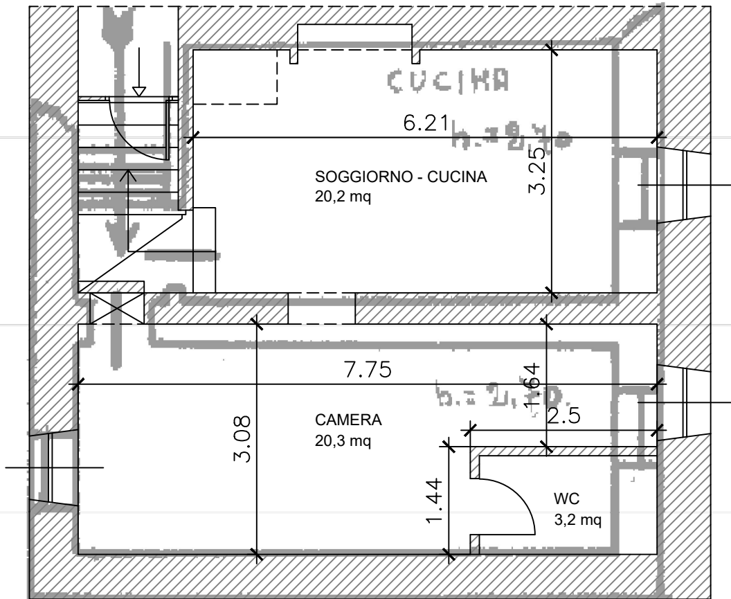
CONFRONTO CATASTALE/RILIEVO
